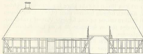
Optegning paa Fæstald og Ladehus bestaaende af 15 Fag.
